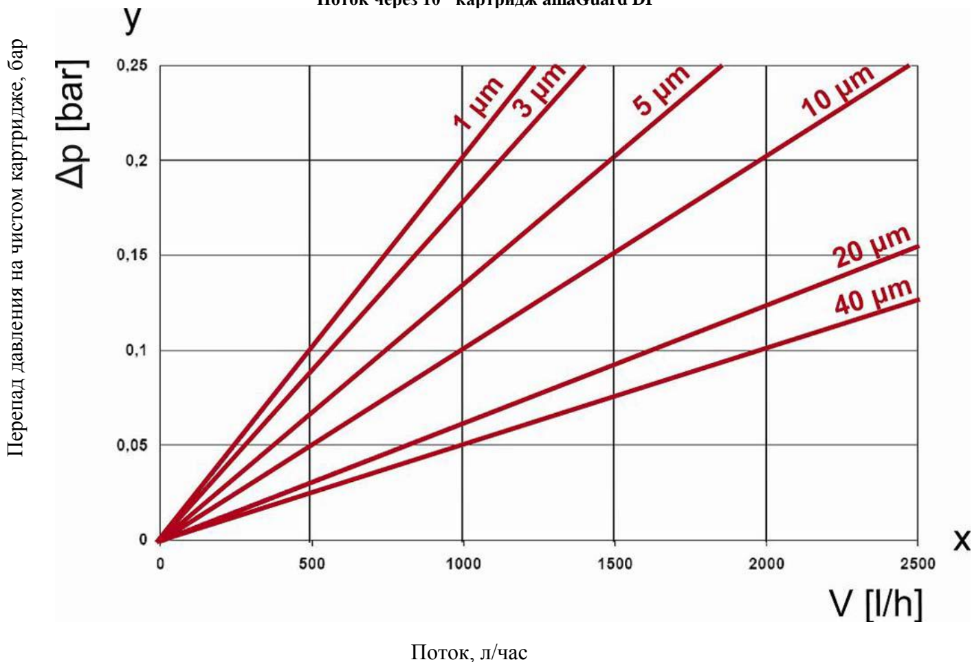
Поток через 10" картридж amaGuard DP
